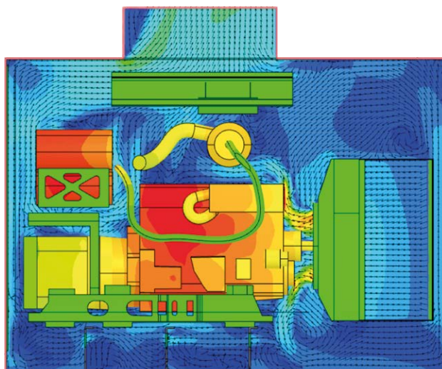
Analyse CFD – Optimisation des flux dès la phase de développement
